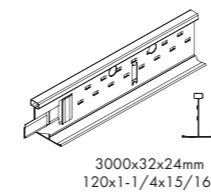
主龙骨 Main Beam
