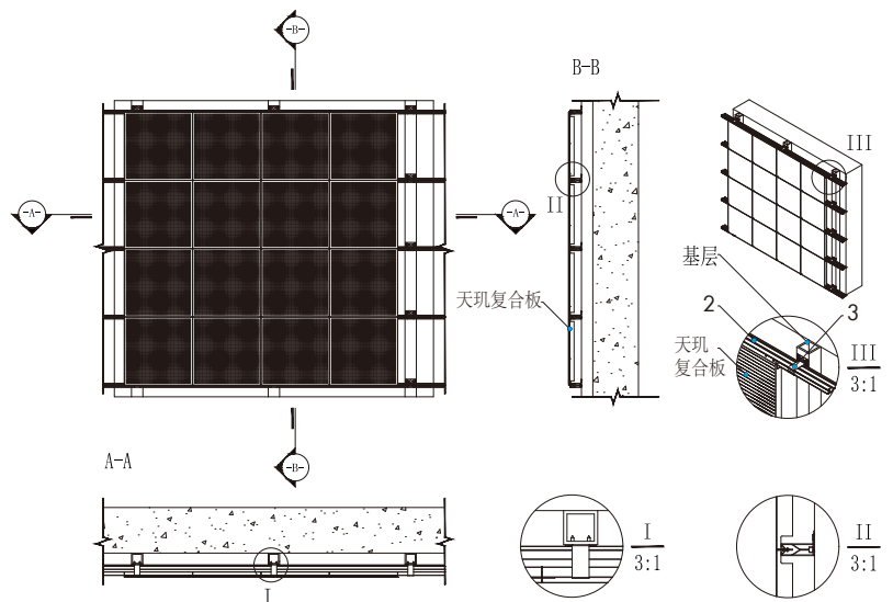
墙面安装示意图
