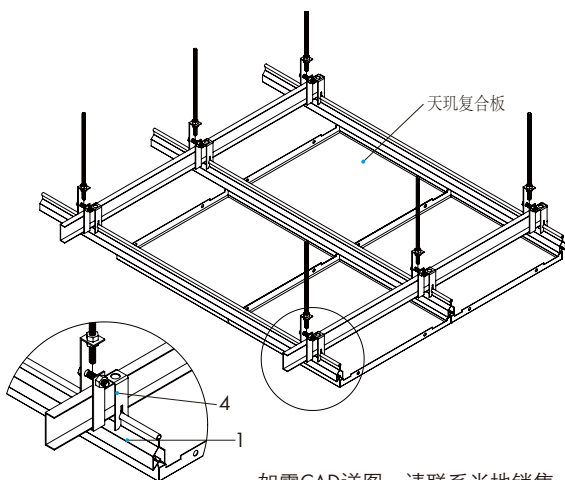
吊顶安装示意图
