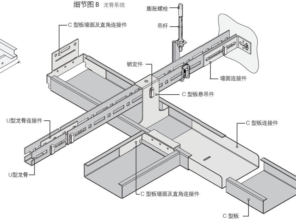
细节图 B 龙骨系统
